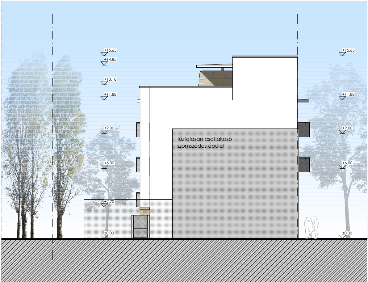
DÉLNYUGATI (TŰZFALI) HOMLOKZAT
