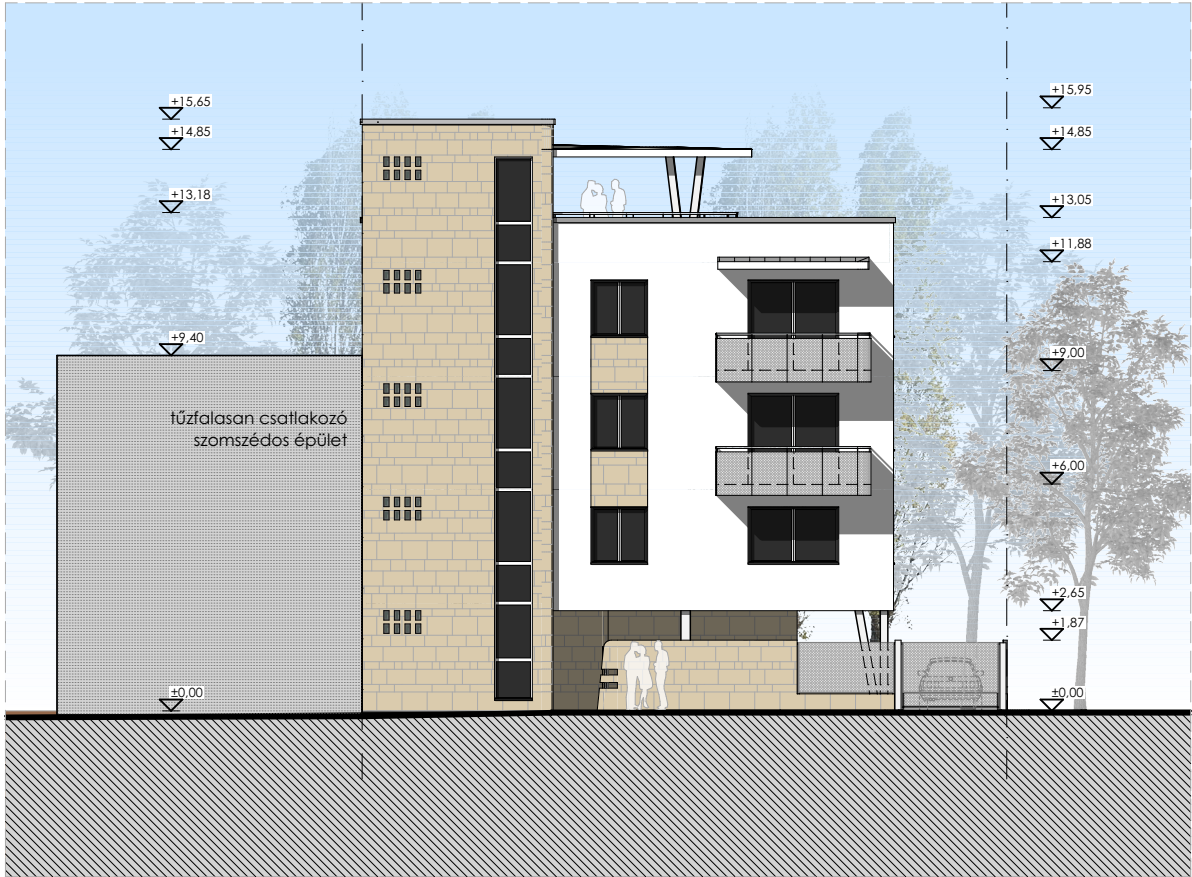
DÉLKELETI (UTCAI) HOMLOKZAT
